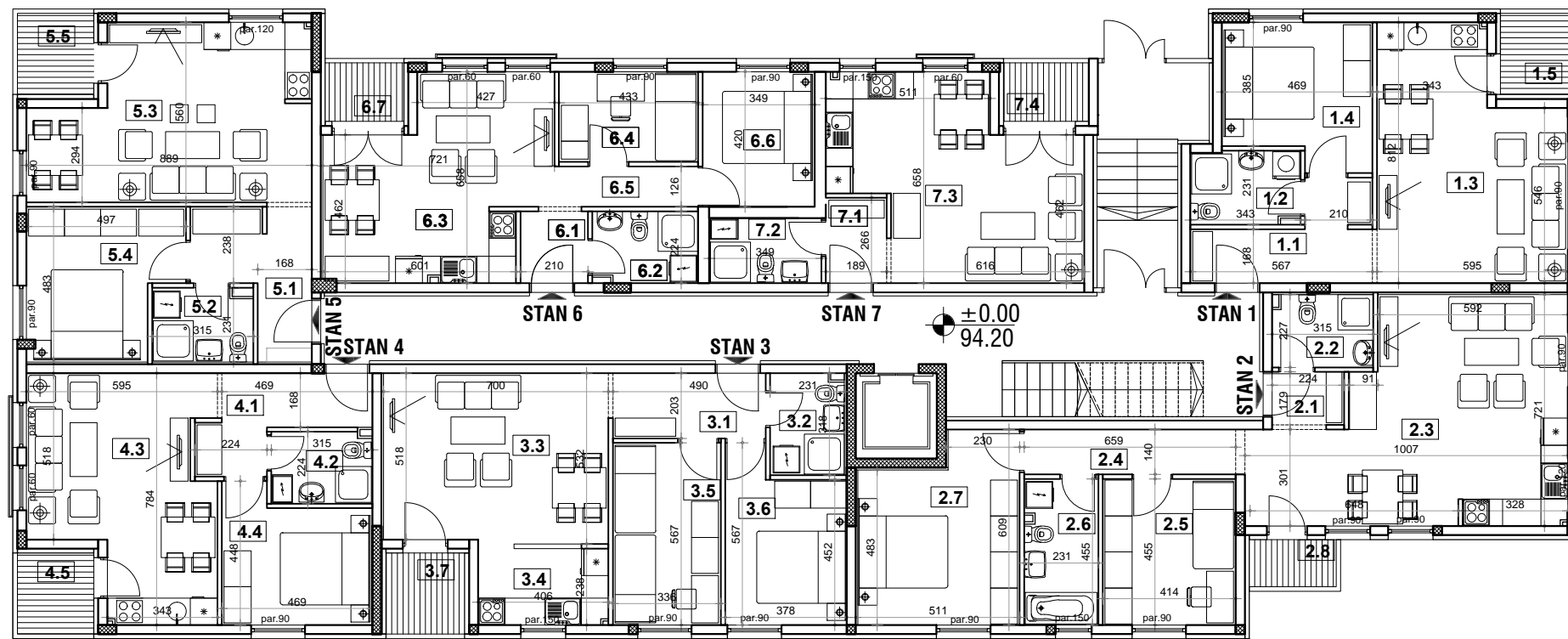
OSNOVA PRIZEMLJA
